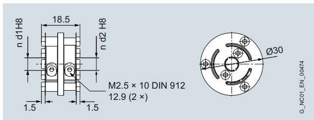
Spring disk coupling, d1 = d2 = 6 \text{ mm}
