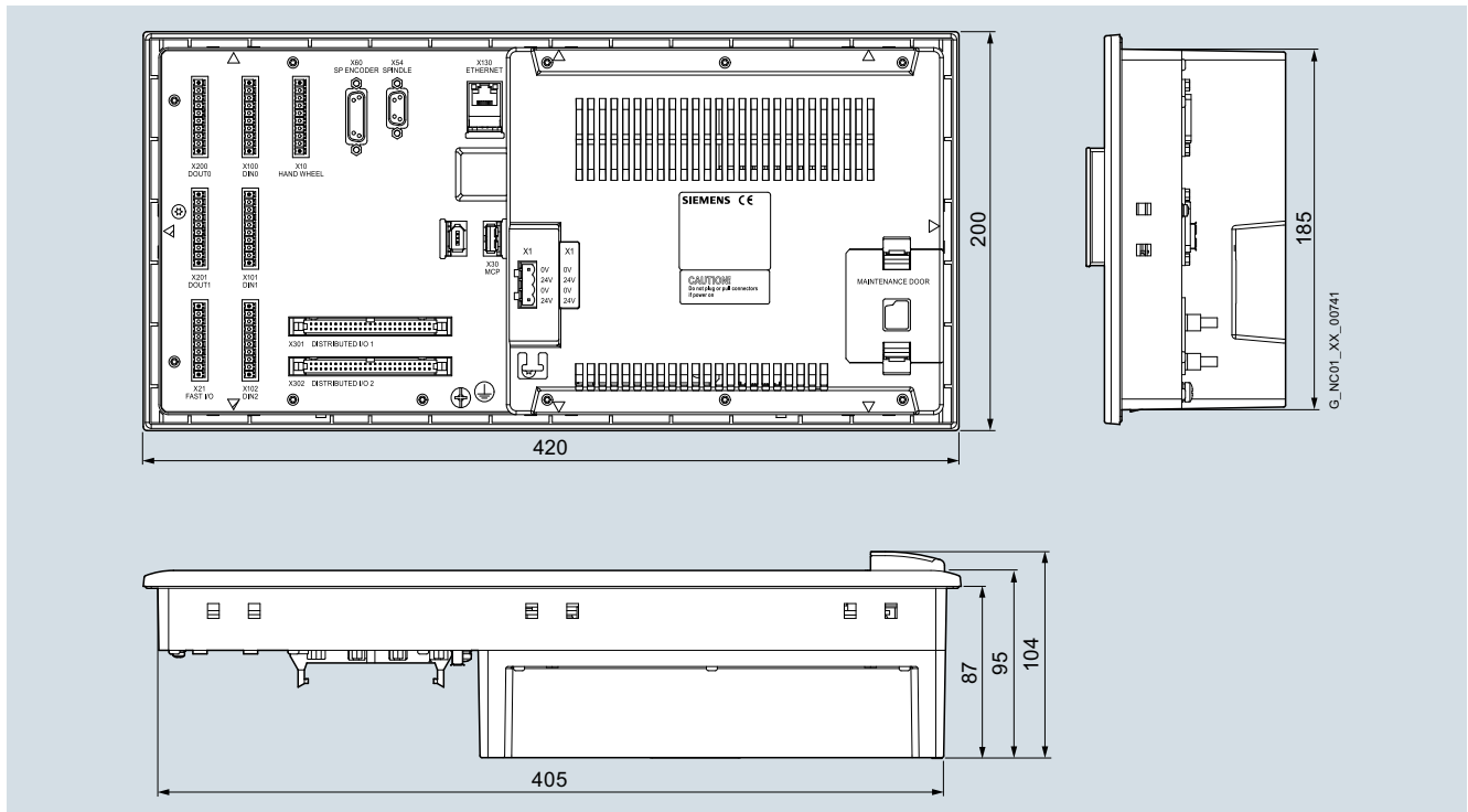
SINUMERIK 808D ADVANCED T/M PPU 161.3 horizontal
